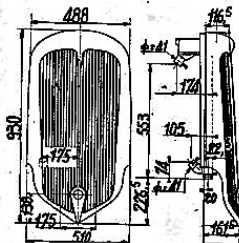
Faisceau de 50 tubes plats quinç., ailettes acier
