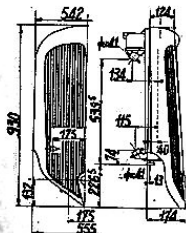
Faisceau de 60 tubes plats quinç., ailettes cuivre
