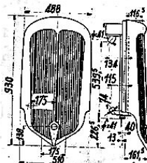
Faisceau de 60 tubes plats quinç., ailettes cuivre
