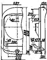
Faisceau 70 (35+5+30) ailettes acier et C. R., tubes plats
