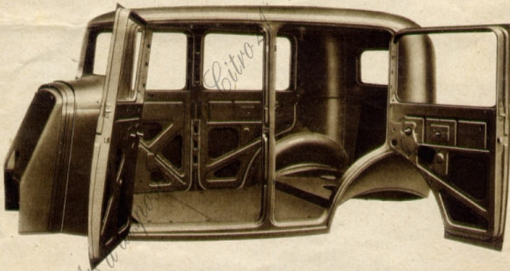
Carrosse d'une carrosserie " Tout Acier Monopiece ". On remarque la solide structure des panneaux et montants entièrement métalliques.
