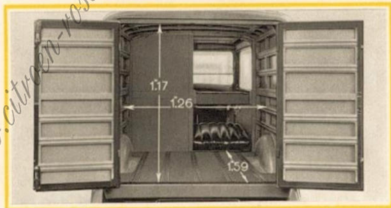
Emplacement disponible pour le chargement dans une 500 kgs
