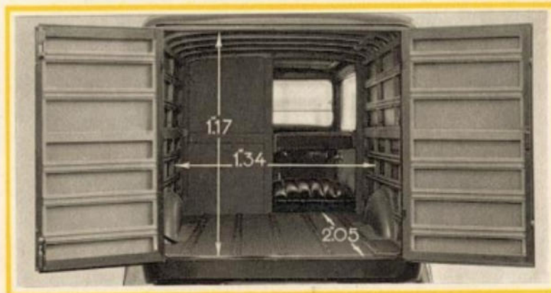
Emplacement disponible pour le chargement dans une 850 kgs
